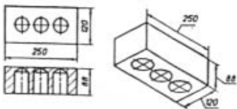
Рисунок А3 — Кирпич 3-пустотный (диаметр отверстий 52 мм, пустотность 15%)
